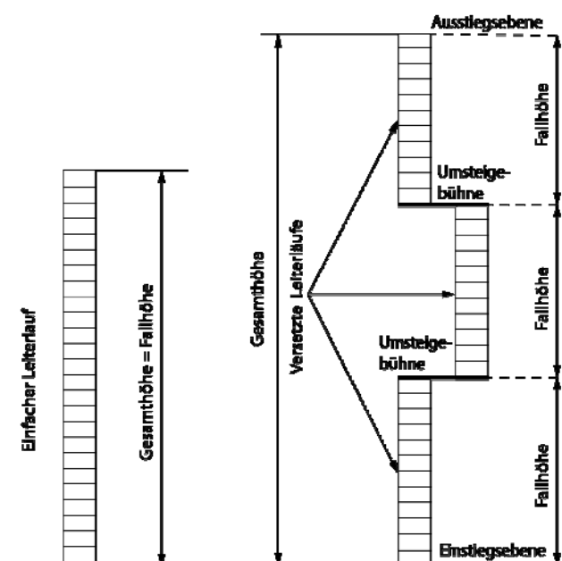
Abb. 1: Beispiel: Fallhöhe, Einstiegsebene
